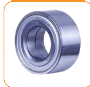
بلبرینگ دوردیفه چرخ جلو ۴۰۵ DAC۴۲۸۲۳۶
